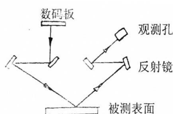
图1 光路图
